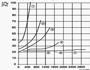
Courbe caractéristique Pertes de charge
